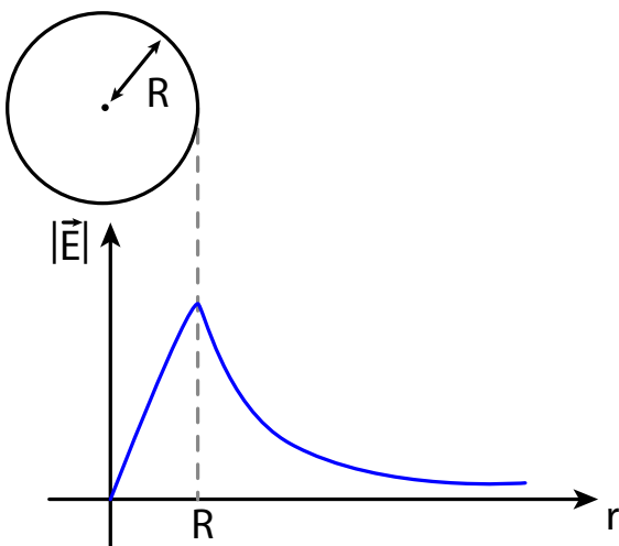
Figura 8 Campo elétrico criado por uma esfera maciça carregada com carga Q.
