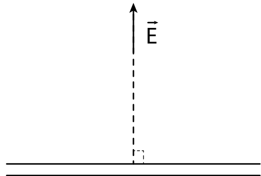
Figura 9 Campo elétrico criado por um filamento muito comprido.
